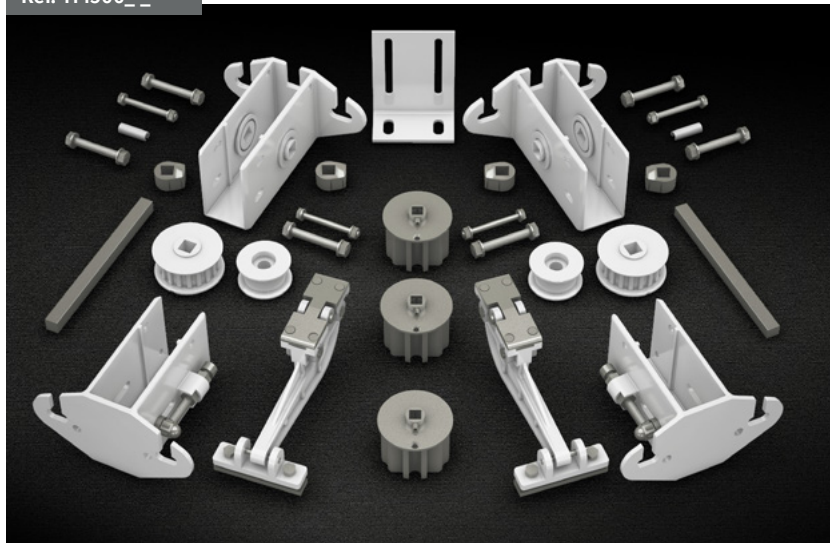
Conjunto Motor Pergo-Sun 80 (incluye escuadras y casquillos) Kit motor Pergo-Sun 80 (plug and valve holders included) Ensemble Moteur Pergo-Sun 80 (équerres et douilles incluses) Conjunto Motor Pergo-Sun 80 (inclui esquadros e casquilhos)
