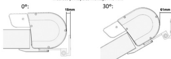
Medidas principales montaje PRO AIR.
