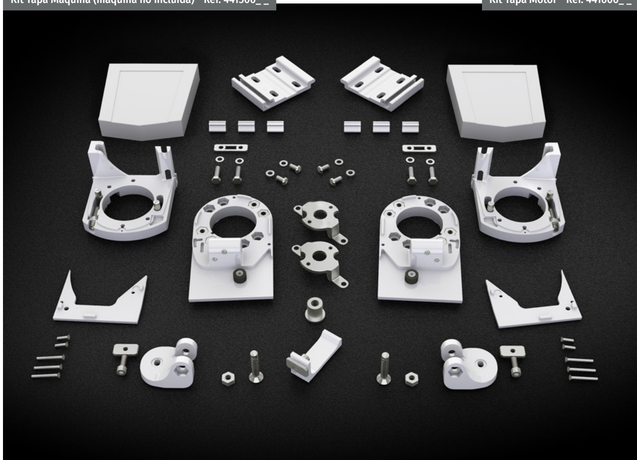
Kit de Accesorios D30 D30 Accessory Kit Kit d'accessoires D30 Kit de Acessórios D30
