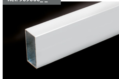
Tubo de Hierro 80 x 40 x 2 Galvanizado y Lacado 80 x 40 x 2 Galvanized and Lacquered iron tube Tube en Fer 80 x 40 x 2 Galvanisé et Laqué Tubo de Ferro 80 x 40 x 2 Galvanizado e Lacado
