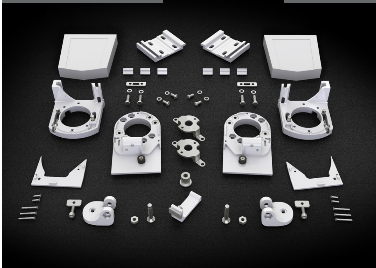
Kit de Accesorios D25 D25 Accessory Kit Kit d'accessoires D25 Kit de Acessórios D25
