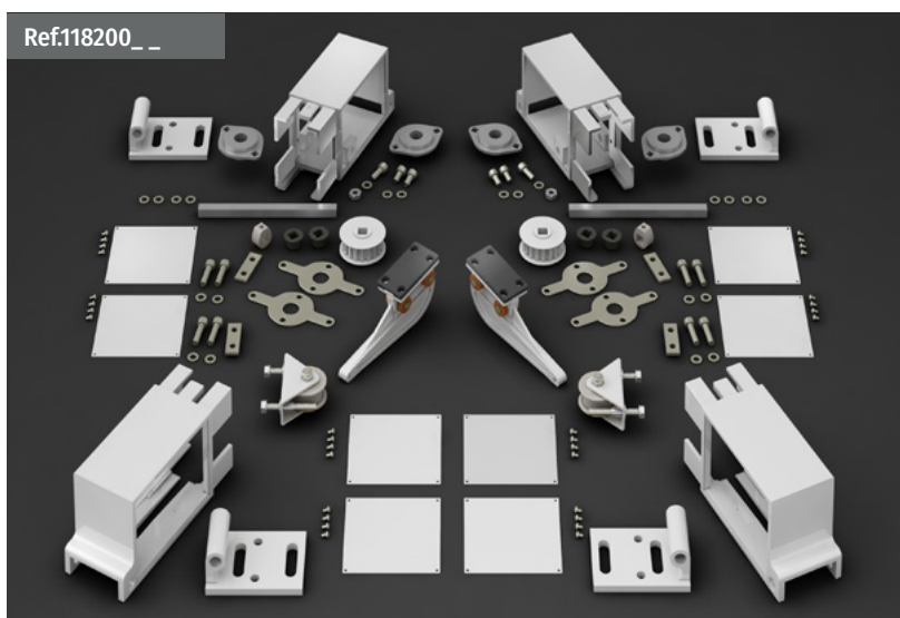
Conjunto Motor 90x96 (incluye escuadras y casquillos) Kit motor 90x96 (plug and valve holders included) Ensemble Moteur 90x96 (équerres et embouts inclus) Conjunto Motor 90x96 (inclui esquadros e casquilhos)
