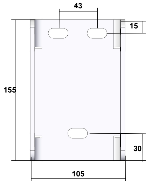
Soporte guía canalón
