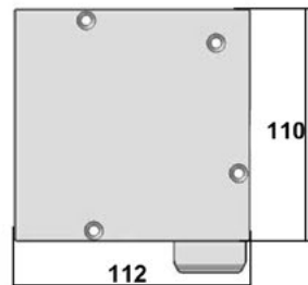
SECCIÓN LATERAL 110 SIDE SECTION 110 PARTIE LATÉRALE 110 SEÇÃO LATERAL 110
