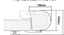
MEDIDAS CON PIE VERANDA PRO AIR
