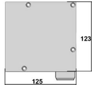
SECCIÓN LATERAL 125 SIDE SECTION 125 PARTIE LATÉRALE 125 SEÇÃO LATERAL 125
