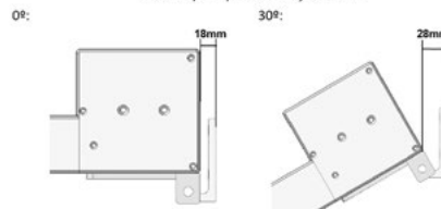
Medidas principales montaje PRO AIR.
